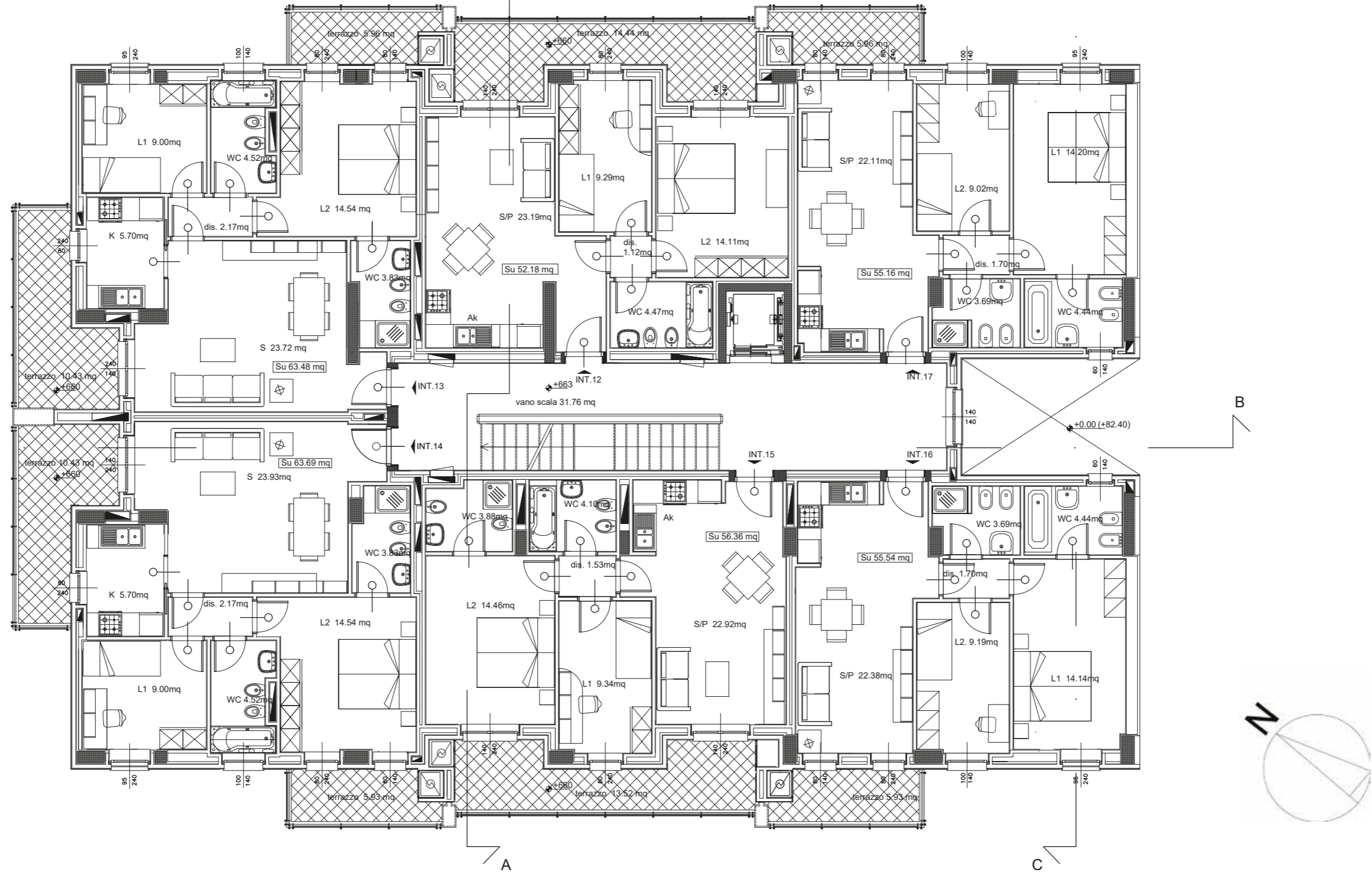
Piano secondo (Pianta fuori scala)
